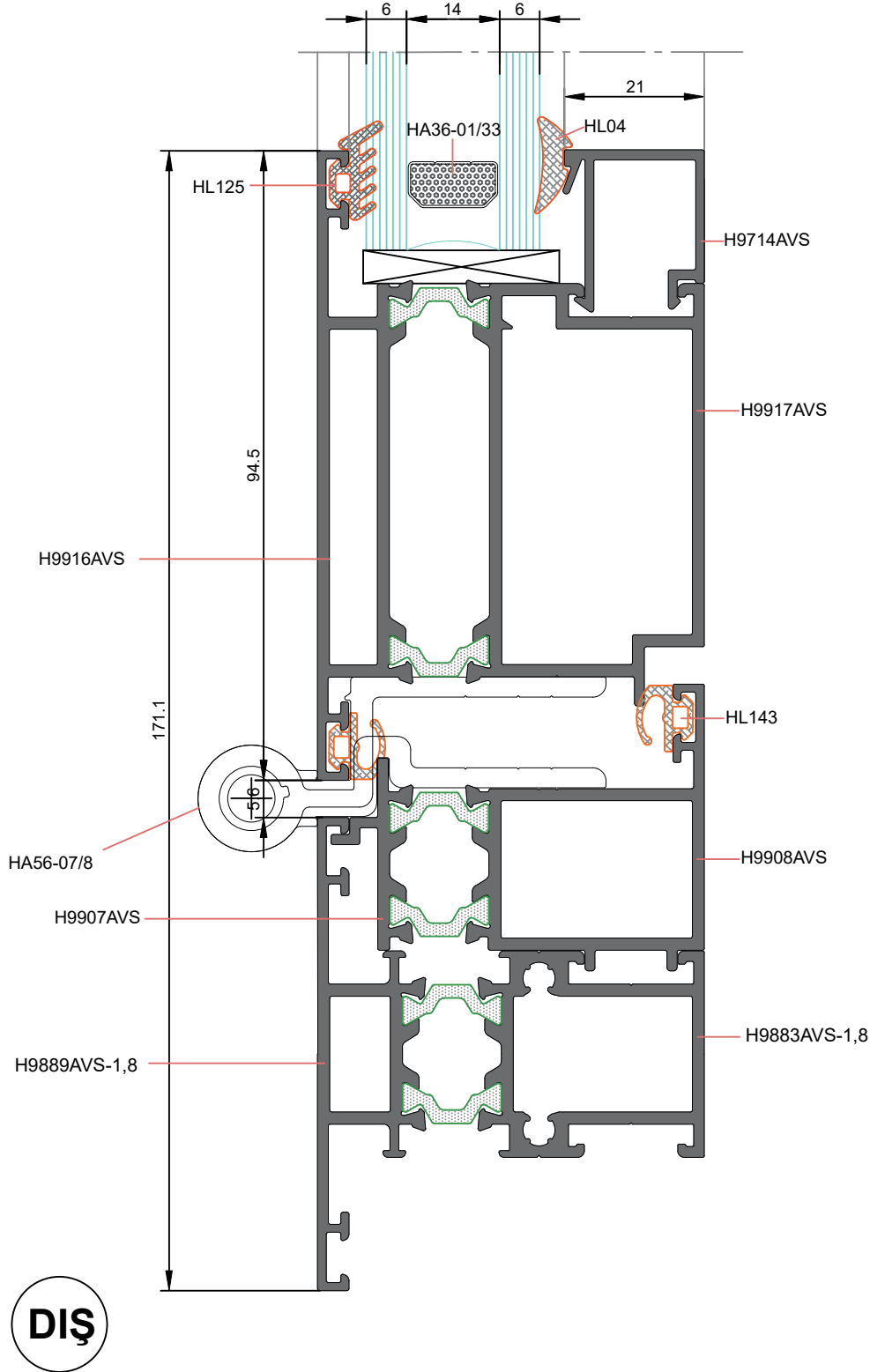
HEMYÜZ DIŞA AÇILIR KAPI
