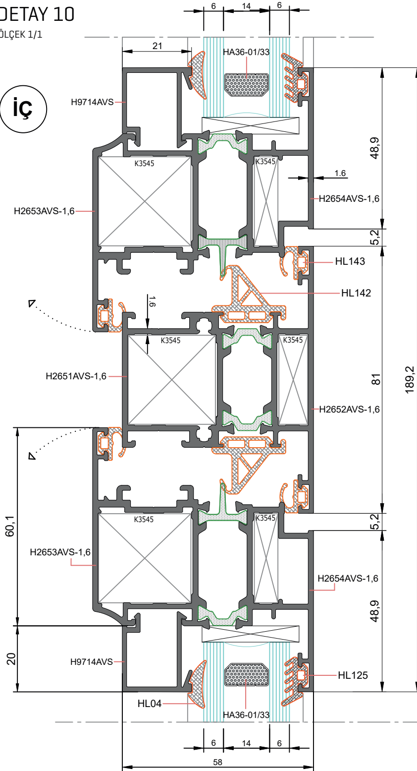
ORTA KAYIT ARALI DETAY
