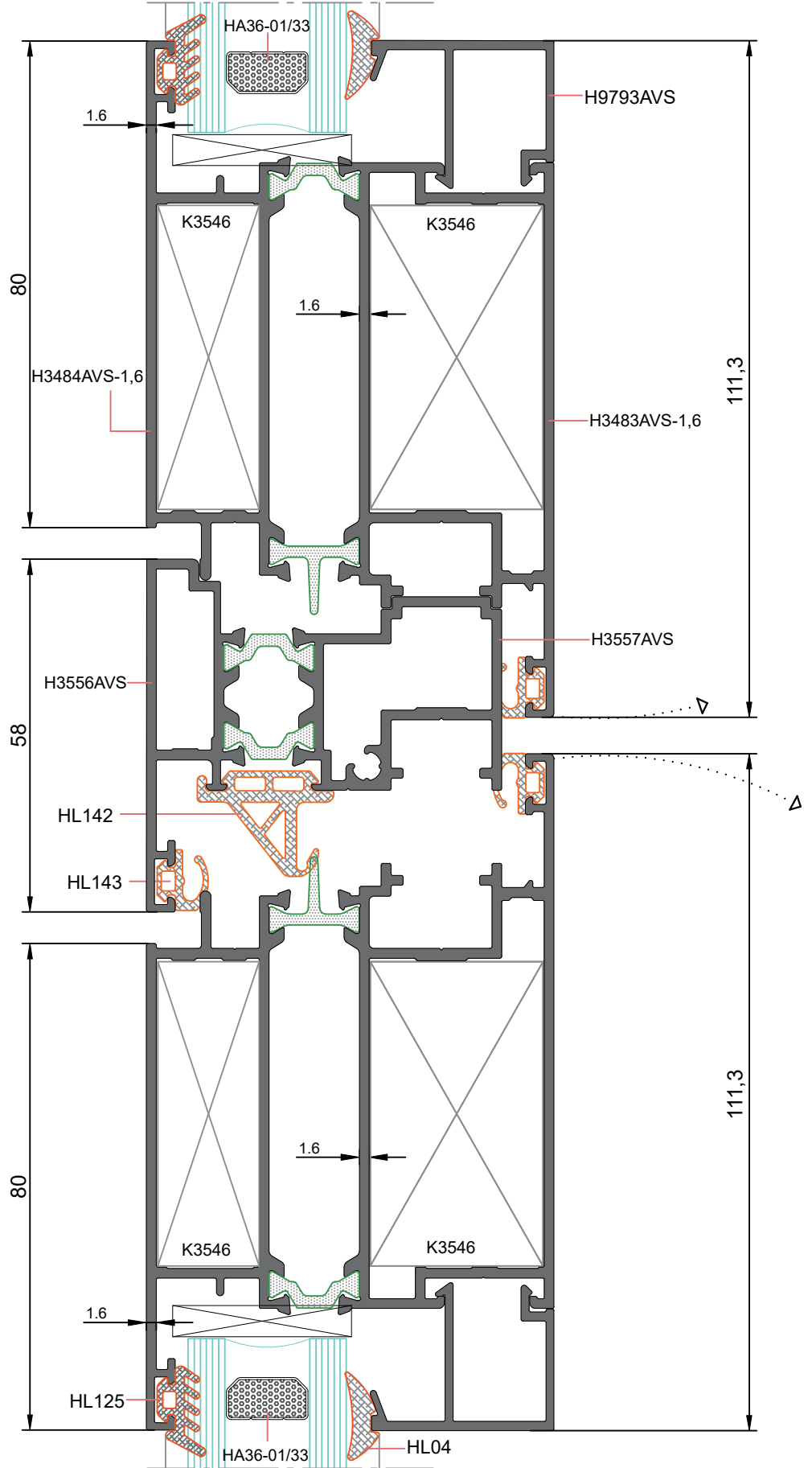
PVC AKSESUARLI DETAY
