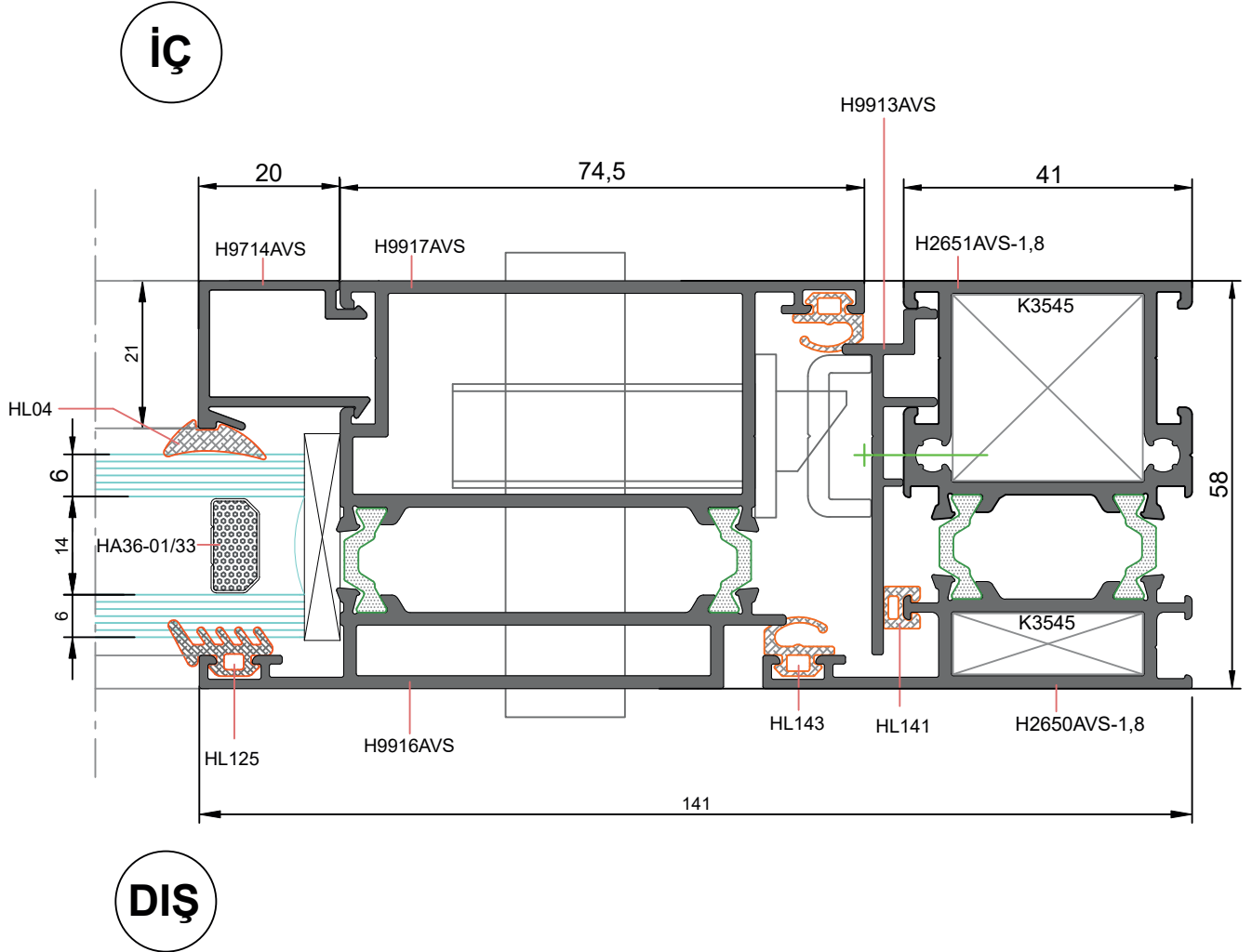
ÇİFT KANATLI HEMYÜZ İÇE AÇILIR KAPI DETAYI
