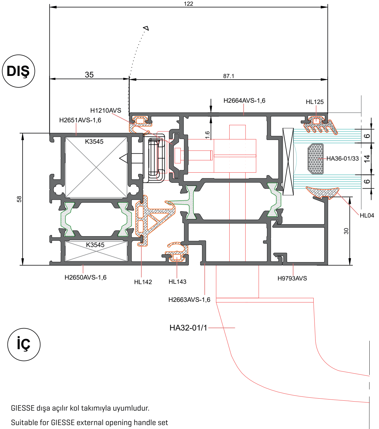
DIŞA AÇILAN PENCERE DETAYI 1.6 LİK
