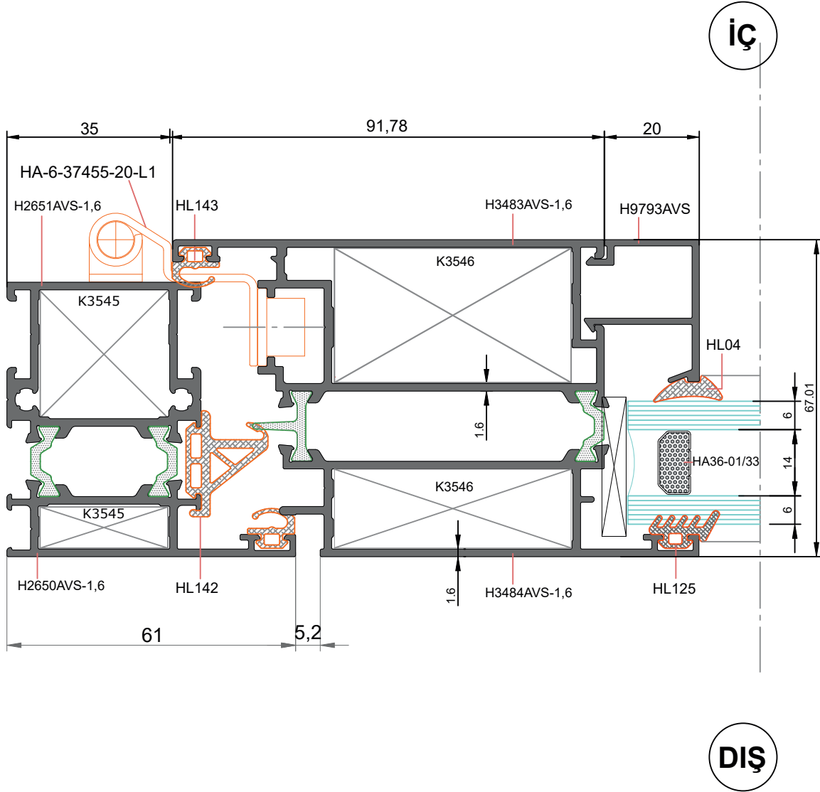
PVC AKSESUARLI DETAY
