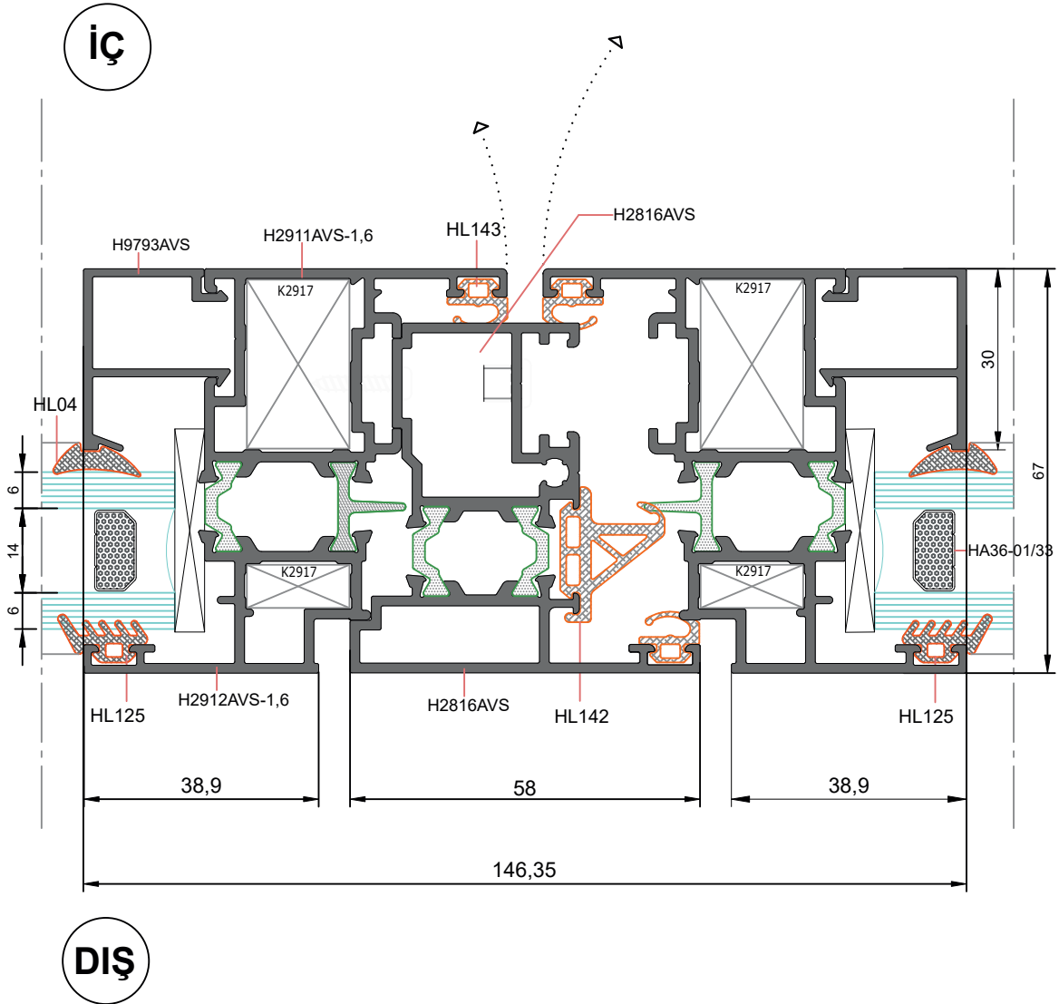
ÇİFT KANAT İÇİN ADAPTÖR DETAYI
