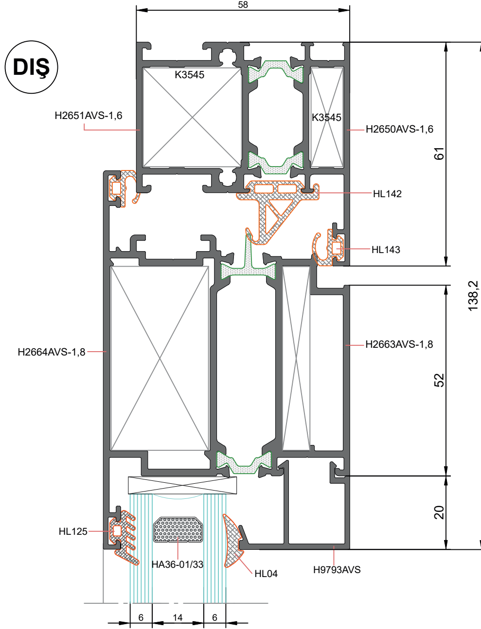
DIŞA AÇILAN KAPI DETAYI TEK KANATLI
