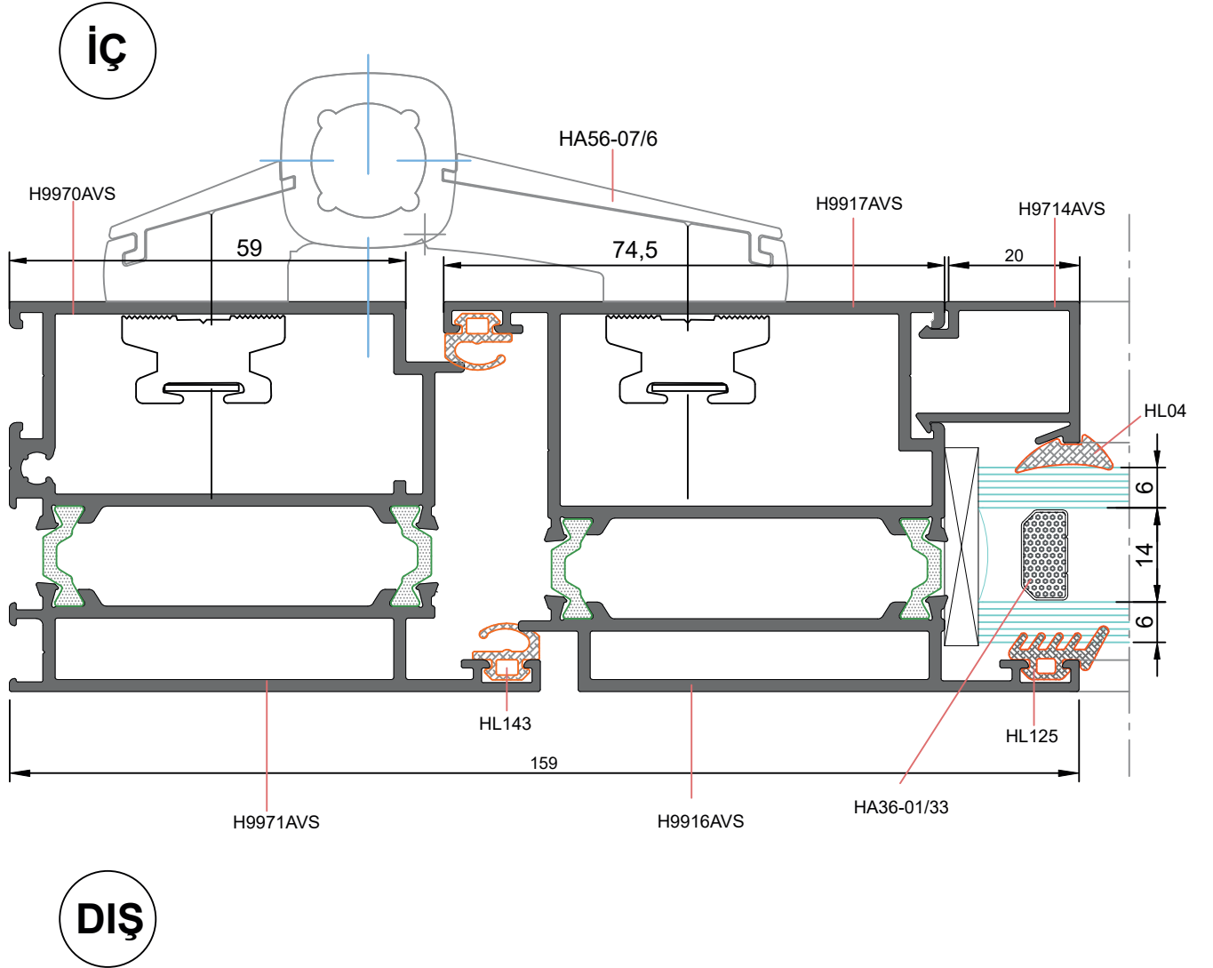
İÇE AÇILIR HEMYÜZ KAPI DETAYI
