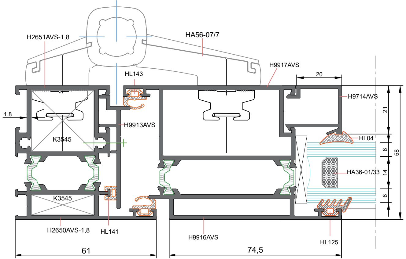
ÇİFT KANATLI HEMYÜZ İÇE AÇILIR KAPI DETAYI
