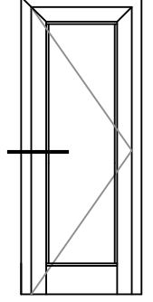
İÇE AÇILIR HEMYÜZ KAPI DETAYI
